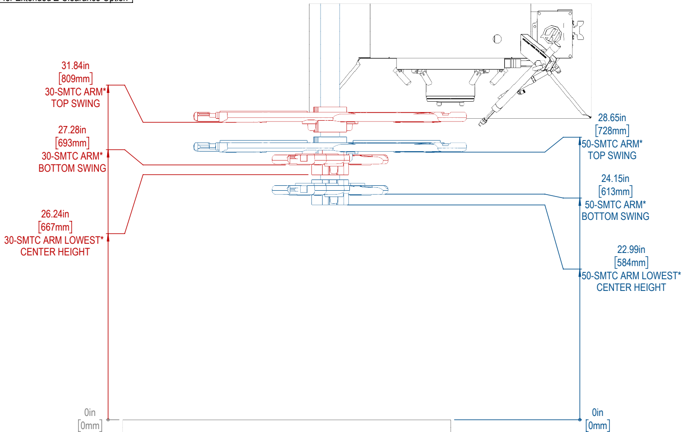
Tool Changer
