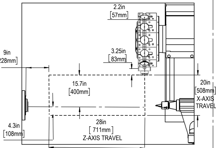
Optional Live Tooling - BMT75 -STRAIGHT
